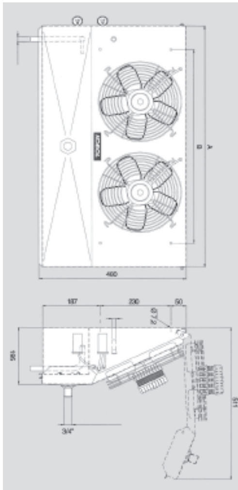
Abmessung MR/MC Serie
